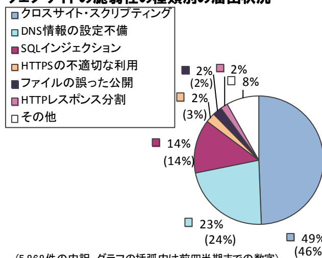
図 2-3. 脆弱性の種類別の届出件数の割合 図 2-4. 脆弱性の種類別の届出件数 (四半期別推移)
