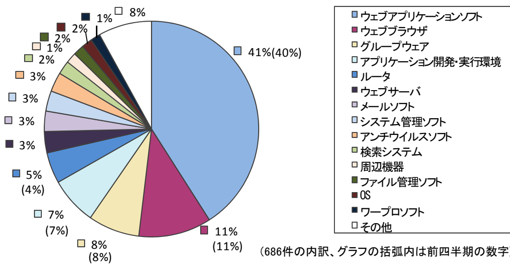
図 1-2.ソフトウェア製品の脆弱性 製品種類別内訳 (届出受付開始から2008年9月末まで)
