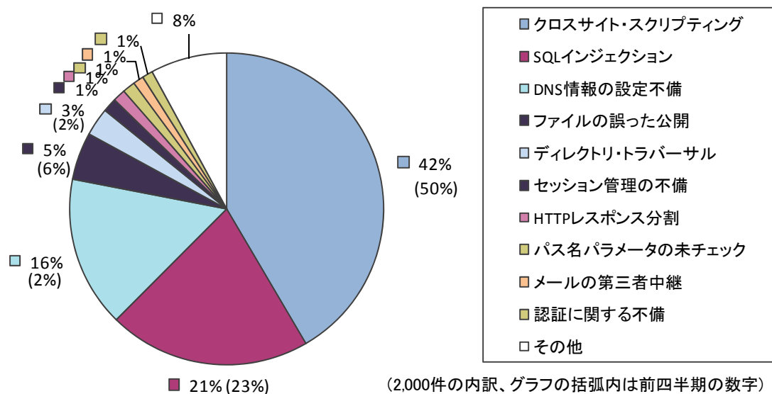
図2-2.ウェブサイトの脆弱性 種類別内訳 (届出受付開始から2008年9月末まで)
